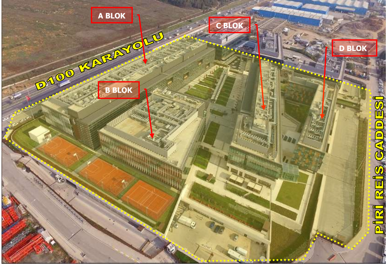
Resim 3. Vaziyet Planı
