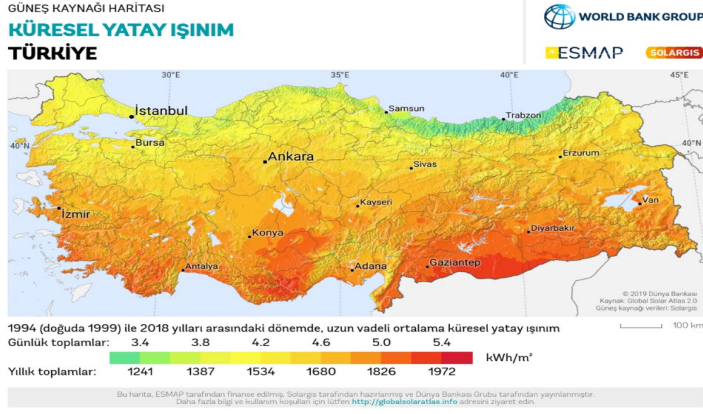
Türkiye Işınım Haritası
