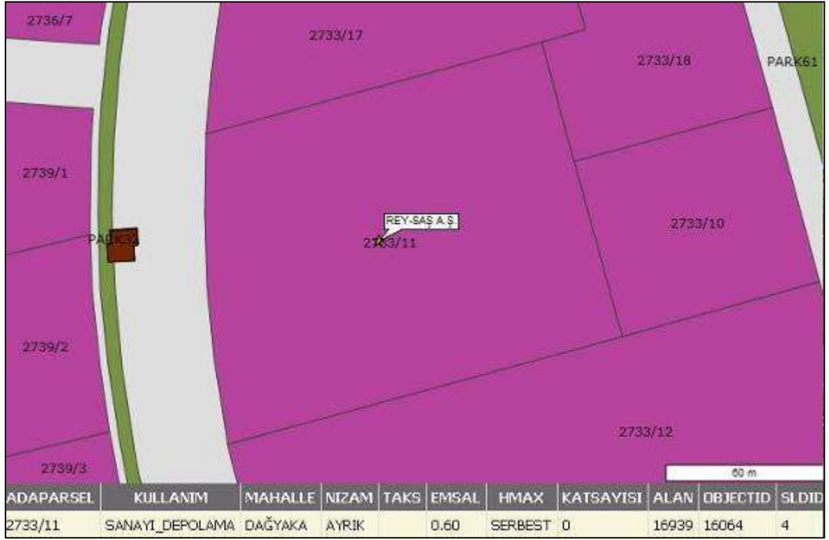
İmar Paftası Örneği (1/1.000)
