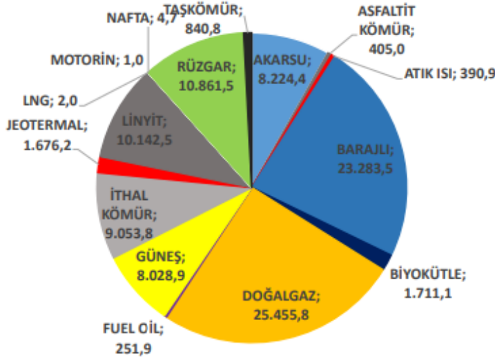
Şekil 5-Türkiye’de elektrik kurulu gücünün kaynaklara göre dağılımı –Mart 2022 Kaynak: TEİAŞ
