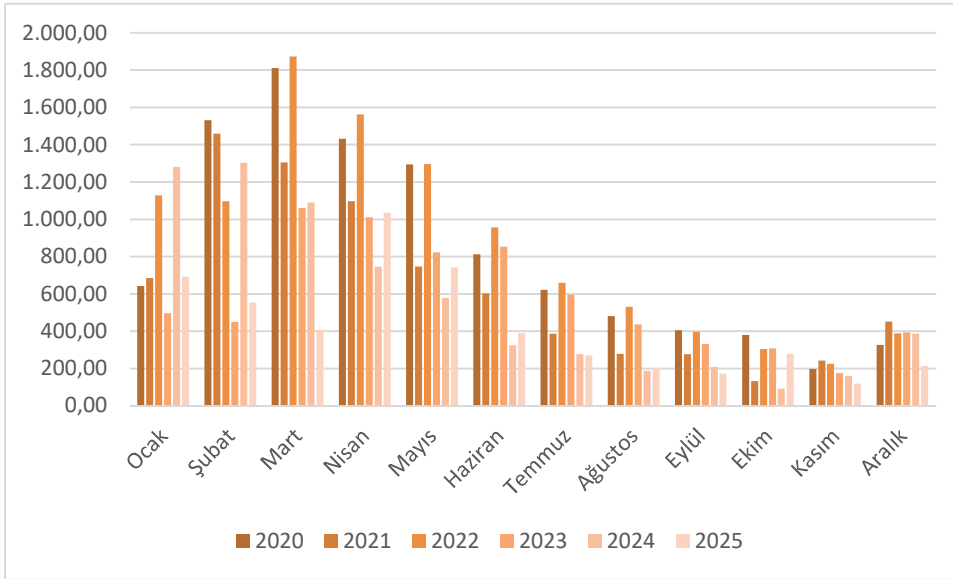
Çukurçay HES Uzun Yıllar Aylara göre Gerçekleşen Üretim Miktar
